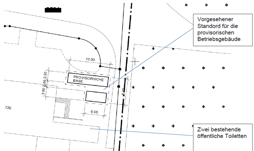
Abbildung 12: Übersichtsplan der Betriebsgebäude und Toiletten, Adventure Coaching & Rope Solutions GmbH, Liestal und die Firma Bolliger + Partner, Chur
